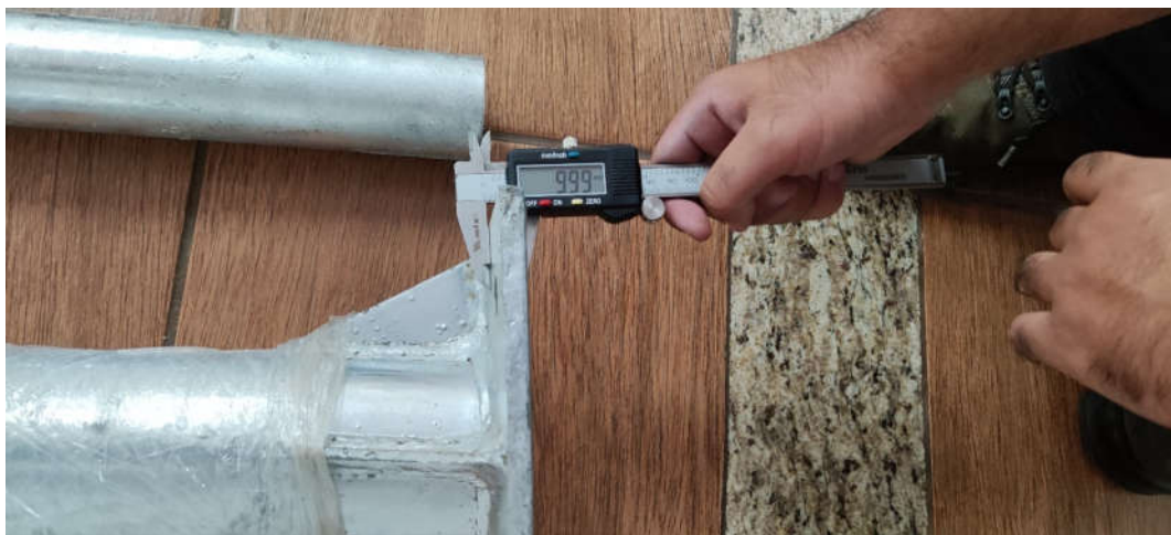
Figura 1. Imagem do Poste Galvanizado 5 metros.
