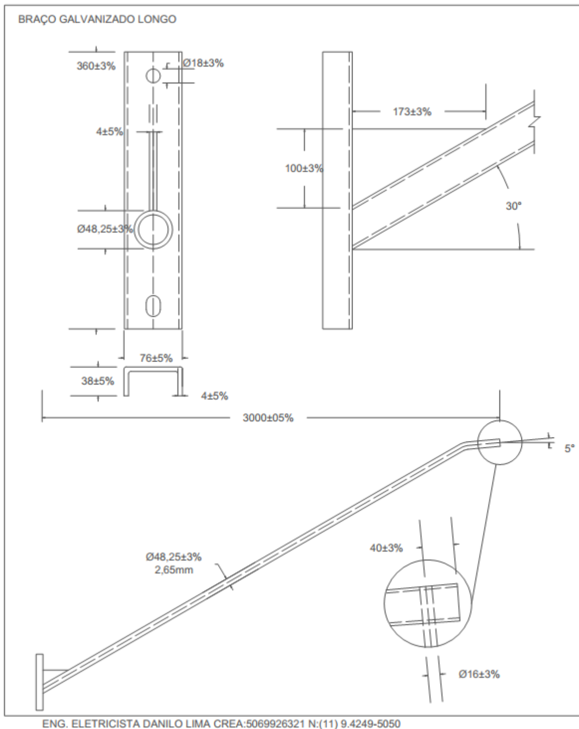
Figura 2 – Braço galvanizado de 3 metros.
