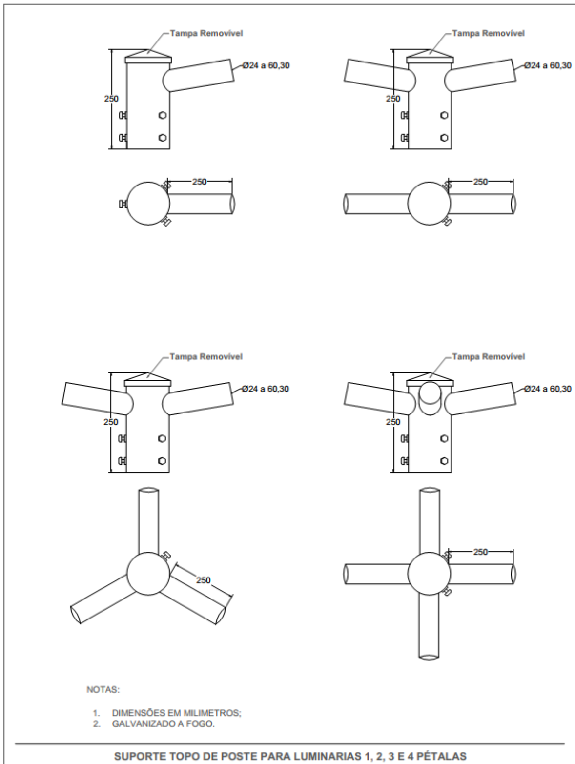
Figura 8 – Suporte topo poste para luminárias 1, 2, 3 e 4 pétalas.
