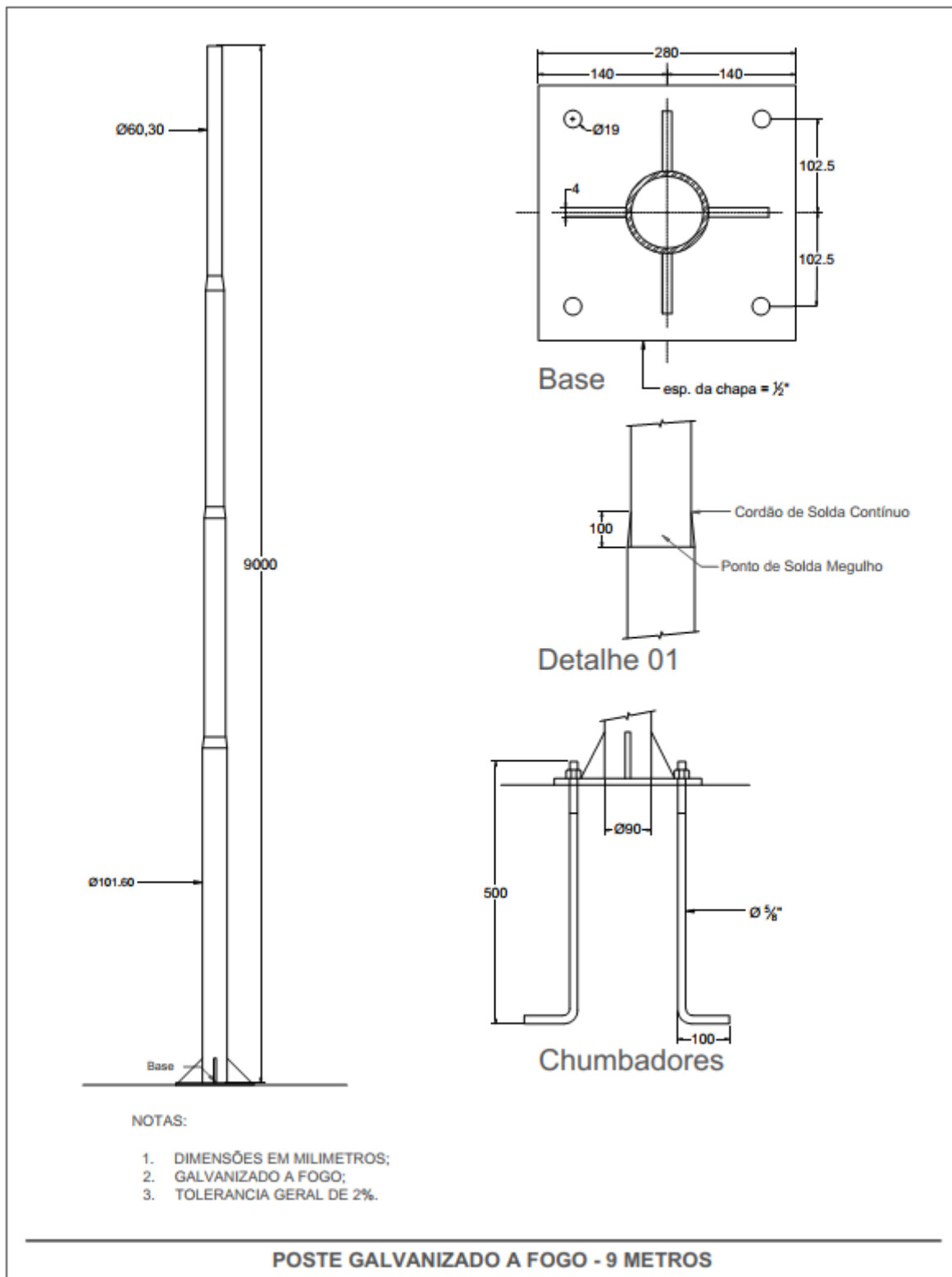
Figura 7 – Poste Galvanizado 9 metros.
