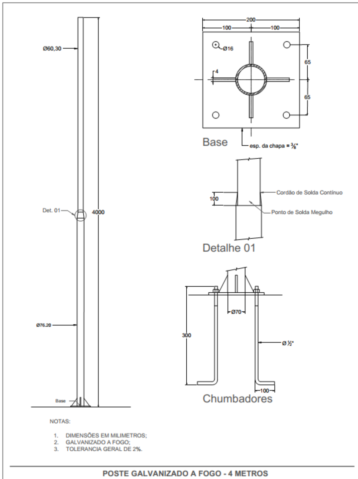
Figura 4 – Poste Galvanizado 4 metros.
