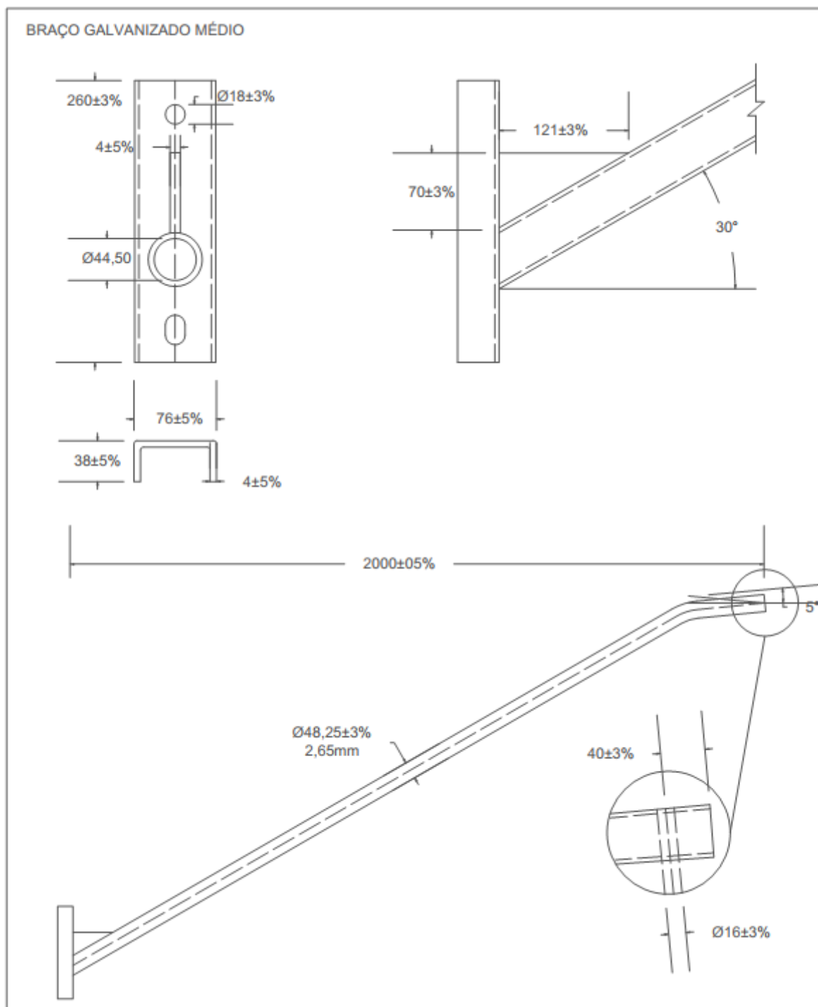
Figura 1 – Braço galvanizado de 2 metros.
