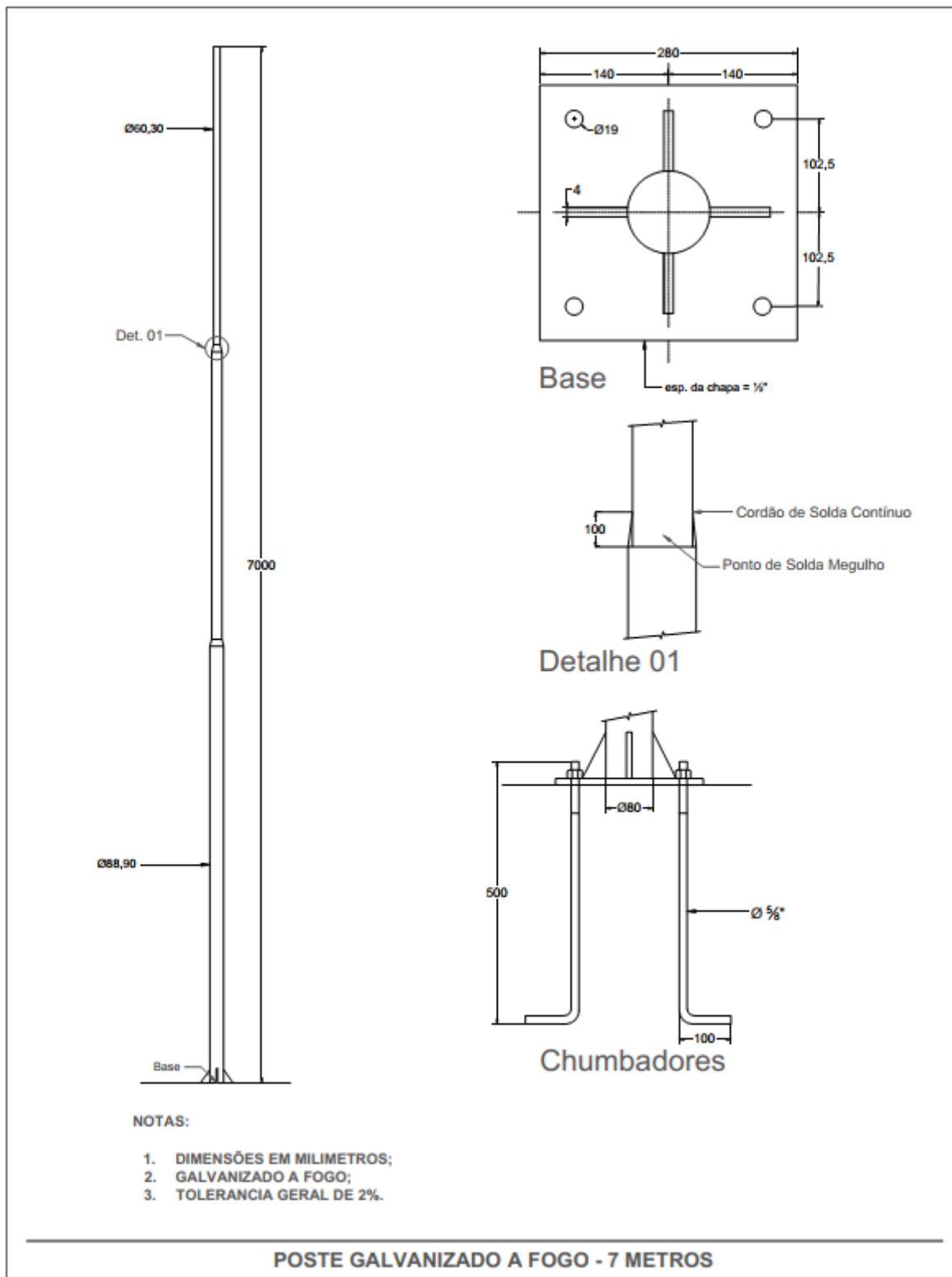
Figura 6 – Poste Galvanizado 7 metros.
