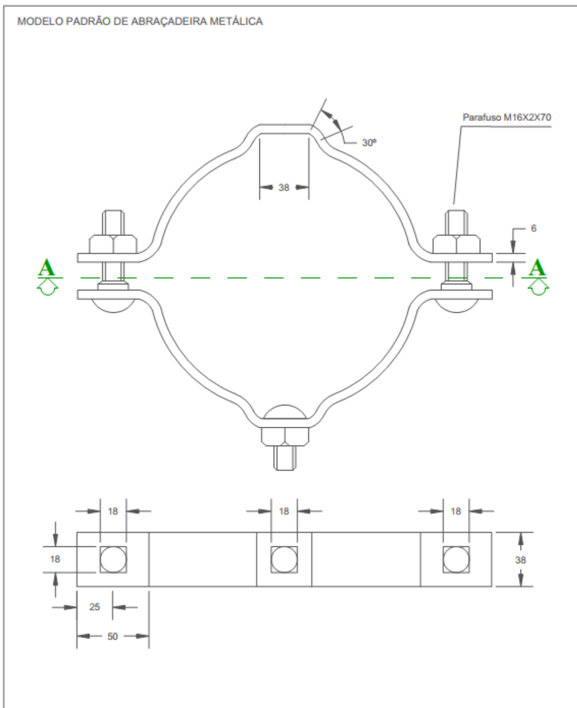
Figura 3 – Modelo das abraçadeiras de aço de 170 a 320mm.
