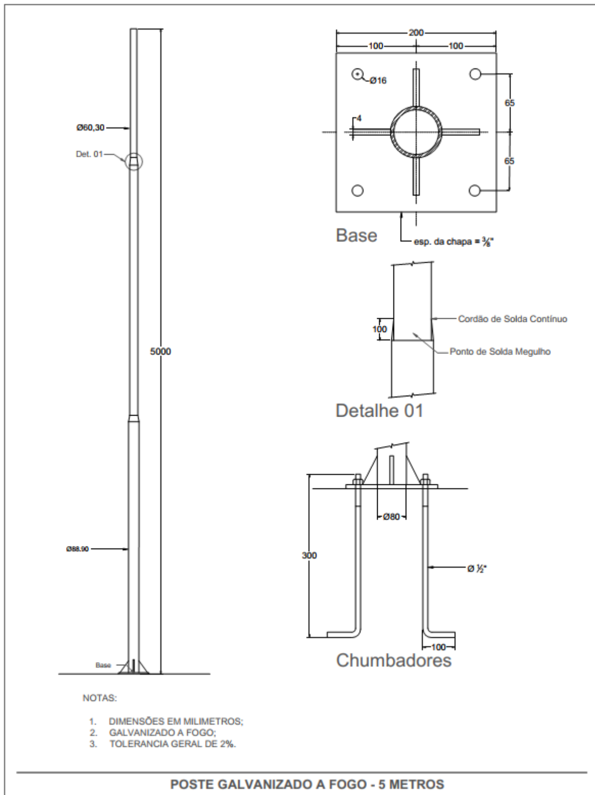
Figura 5 – Poste Galvanizado 5 metros.
